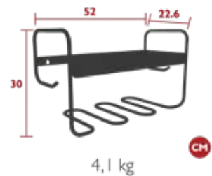
Stahldrahtgestell Regal aus Stahlblech 2-hacken an jedem ende zum am-und Aufhänger verschiedener gegenstände Wandbefestigung (schrauben nicht inbegriffen)
